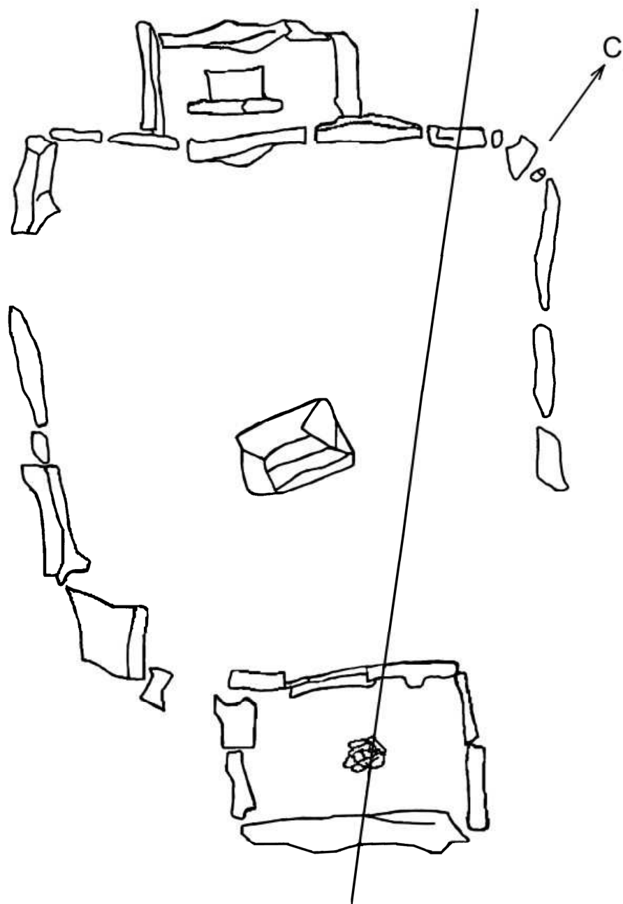
Табл. II. Могильник ДА-I-2. Основа оградки с пристройкой, план
